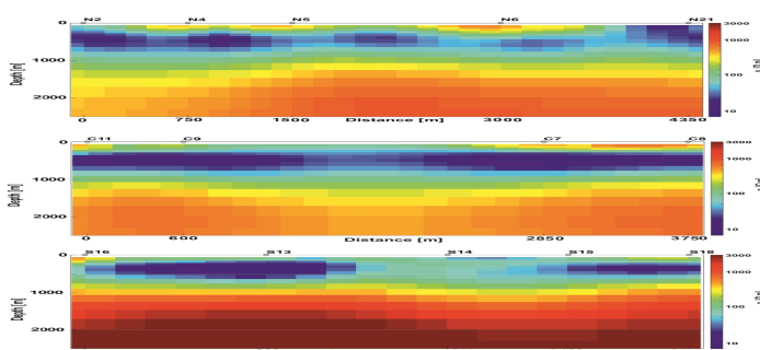
شکل ۳- مدل سازی دوبعدی داده های AMT در امتداد پروفایل ها
