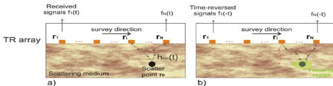
شکل 1. اصول روش TR، الف: پراکنش موج ارسالی در یک ناهنجاری ب: سیگنال‌های باز گسیل شده مصنوعی (سانتوس، 2017).
